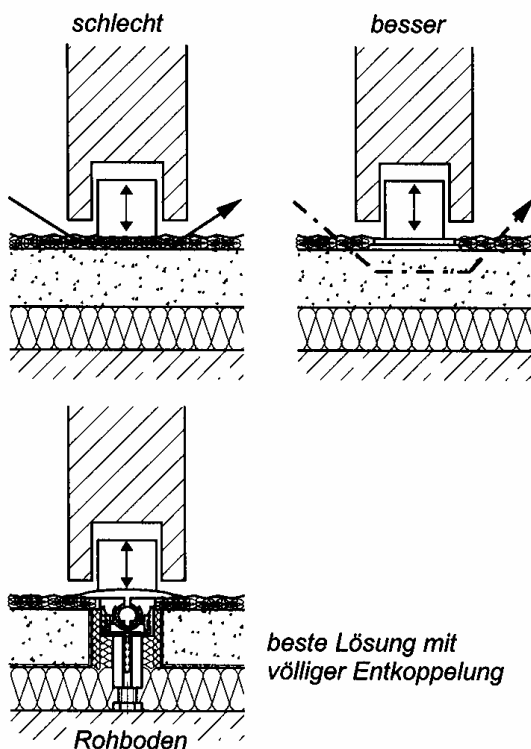
Bild 11 Schallübertragungswege u. Entkoppelungsmaßnahmen im Fußbodenanschlussbereich
