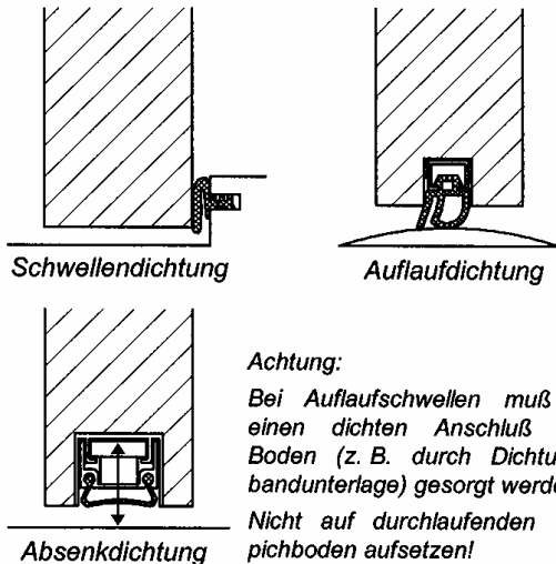
Bild 10 Abdichtungsmöglichkeiten zwischen Tür und Fußboden
